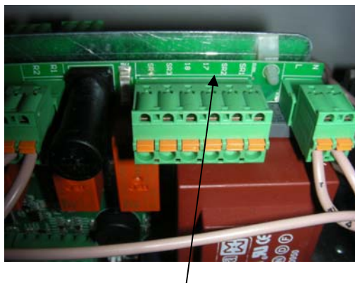
Выходы датчика SR1 и SR2, а также 17 и 18 печатной платы
